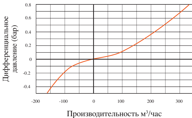
График пропускной способности клапана в кинетическом режиме
